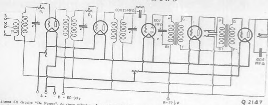
Diagrama del circuito "De Forest", de cinco válvulas. Las unidades "E-1" y "E-2" se llaman "Dispositivos anti-entradas". Estos dispositivos regulan las oscilaciones del circuito. La "Tierra" va conectada al polo negativo de la batería "A". Las conexiones de la placa y de la rejilla deben ser lo más cortas posible, mientras que las demás conexiones de las baterías puedan formar un solo cable.
